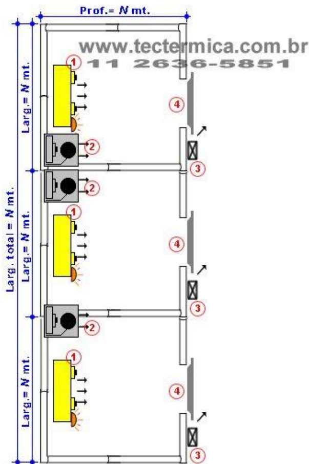
Referência do layout: Camara fria tripla, montada lado a lado
