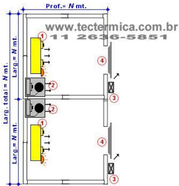
Referência do layout: Camara fria dupla, montada lado a lado
